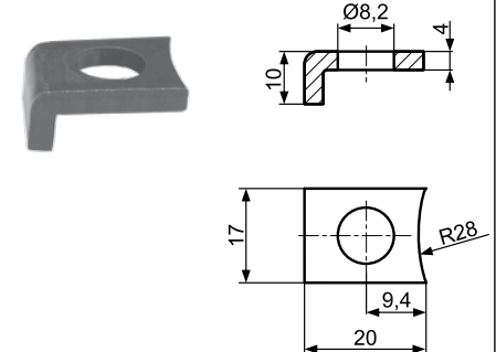
Zaczepek RCL Clamp RCL
