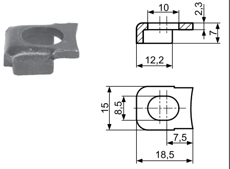
Zaczepek RCC dla tulei BEB Clamp RCC for bush BEB
